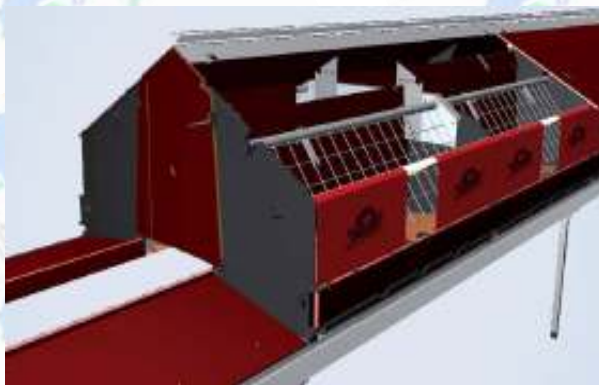
PONEDERO AUTOMATICO (DETALLE DEL NIDO)
